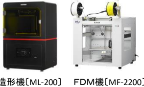
光造形機〔ML-200〕 FDM機〔MF-2200〕
