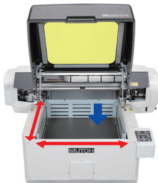
最大メディアサイズ / 重量 594 (D) x 483 (W) x 150 (H) mm / 6kg
