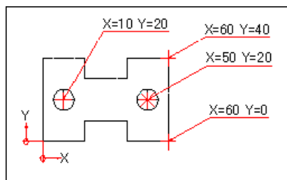
通常形式の座標寸法
