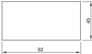
パネルカット寸法
